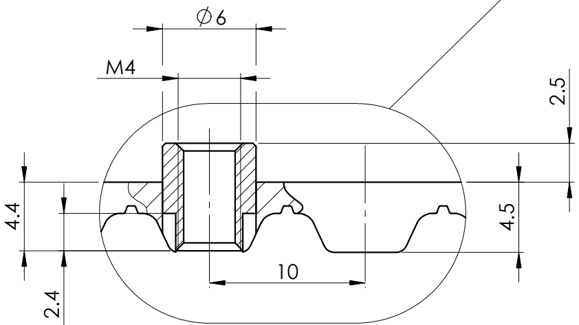
DETTAGLIO B SCALA 3 : 1
